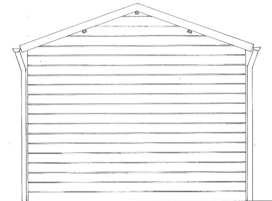
Voorgevel
